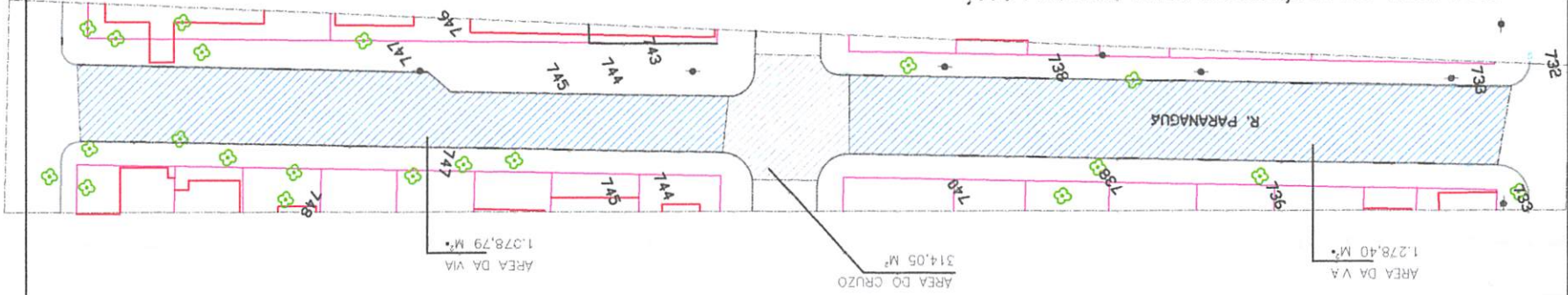
ESC. 1/25 PROJETO GEOMÉTRICO (RUA PARANAGUÁ - TRECHO 01)
