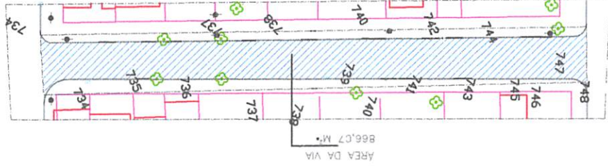
ESC. 1/25 PROJETO GEOMÉTRICO (RUA PARANAGUÁ - TRECHO 01)
